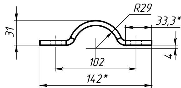
Поз.4 (Полухомут)
